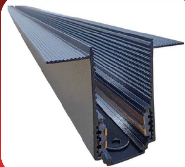
*54x45.7mm maqnit rels alüminium profil *Eni: 25 mm *3 metrəlik
